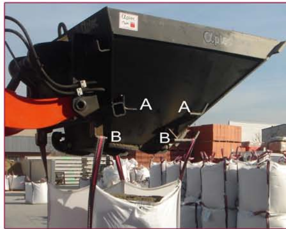
▲ Puntos de anclaje opcionales para otro tipo de sacos (A: fijaciones estándar, B: fijaciones opcionales) Optional fixing points for other bags (A: standard fixing points, B: optional fixing points)
