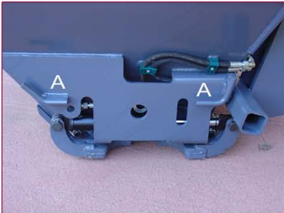
▲ Puntos de anclaje estándar (A) para Big Bags. Standard fixing points (A) for Big Bags.
